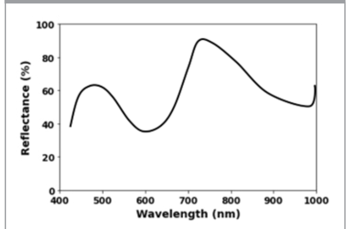
↑ a) Longueurs d'onde de PanCam comparées aux données multispectrales, b) Exemple de données hyperspectrales
