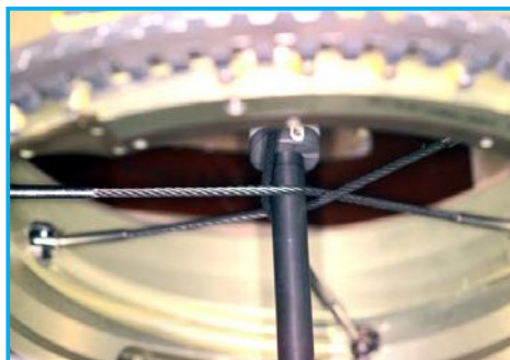
Les collets sont refermés autour de l'axe de fixation d'un grappin sur le bras robotique.
